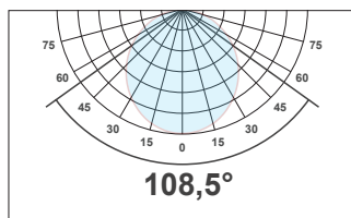
DIFUSOR Opalino
